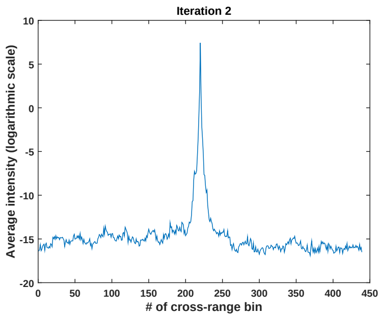
Kuva 3.5: Etäisyys suunnan yli laskettu keskiarvo intensiteettikuvasta 3.3 (toinen iteraatio).
