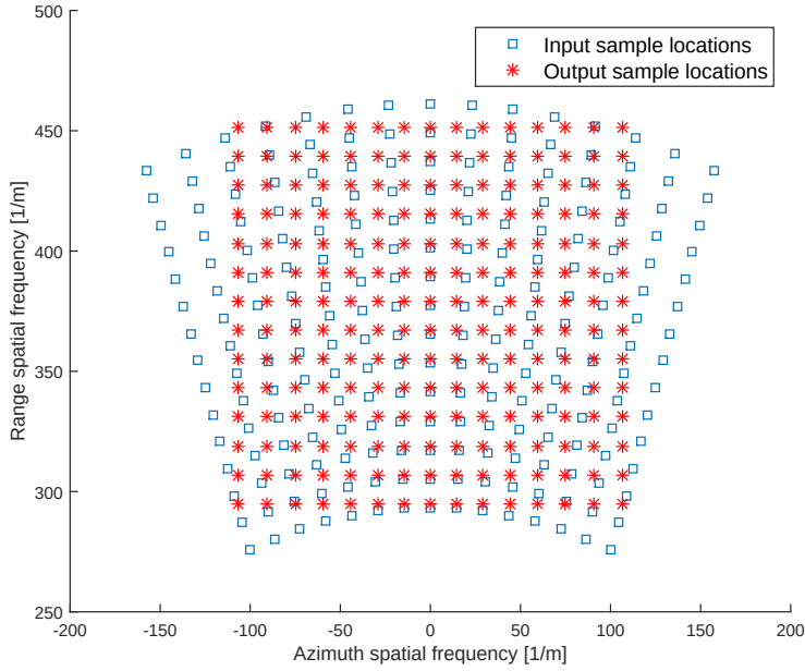
Kuva 1.3: Näytepisteet napakoordinaattimuodossa ennen uudelleennäyteistystä (siniset laatikot) sekä uudelleennäytteistyksessä käytetty karteesinen ruudukko (punaiset tähdet). Pystyakselin muuttuja on k_x ja vaakakselin k_y .
