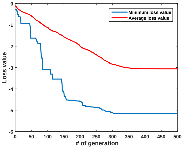
Kuva 2.11: Hiukkasparvioptimoinnin konvergoituminen, kuvassa näkyvät populaation paras kohdefunktion arvo (sininen) ja koko populaation keskiarvo (punainen). Kohdefunktiona on (2.3).
