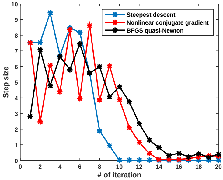
Kuva 3.24: Kunkin iteraation askelkoko eri algoritmeille.
