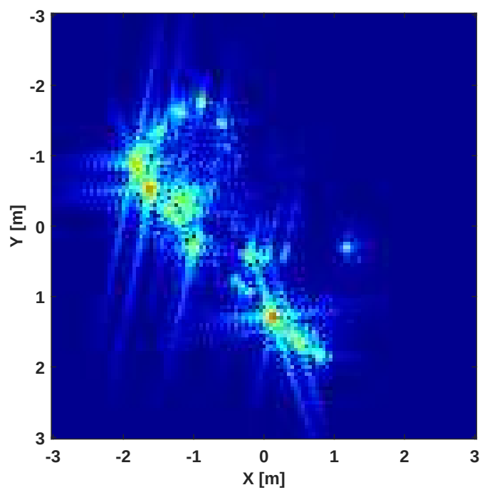
Kuva 4.11: Idealisesti fokusoitu, takaisinprojektiolla laskettu ISAR-kuva.
