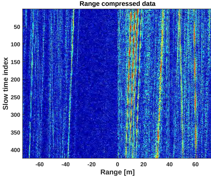
Kuva 1.4: Etäisyyskompressoidun tutkadatan intensiteetti logaritmisella skaalalla.
