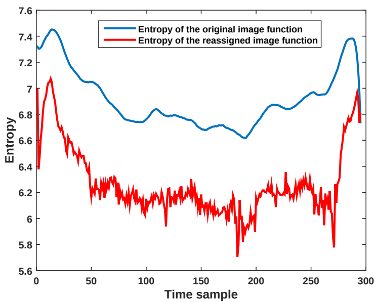
Kuva 4.10: Intensiteettikuvien entropia ennen uudelleensijoitusta ja uudelleensijoituksen jälkeen.
